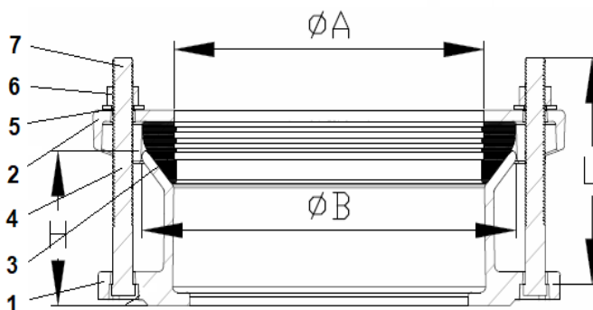
Рис.3. Муфта/адаптер ПФК
